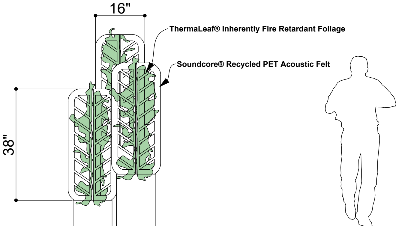
① ELEVATION 1
